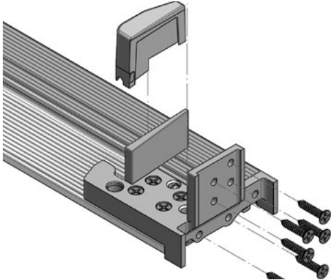
Schwellenhalter (SH...) aus Kunststoff inkl. Falzdichtung und Schwelldichtung
