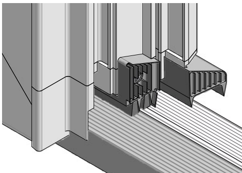
Stulpabdichtung (STK...)* aus Weichkunststoff | inkl. Edelstahlschrauben
