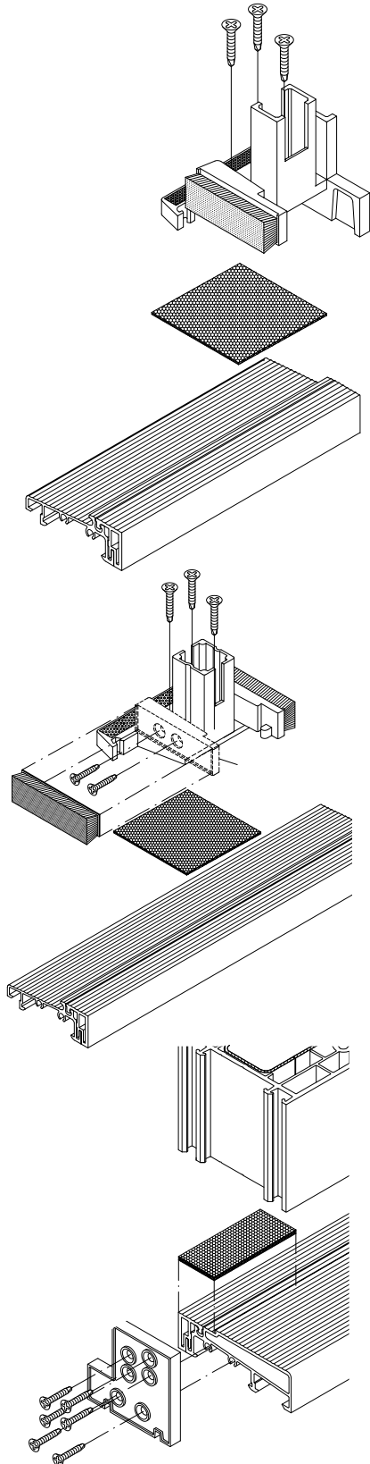
Schwellenhalter (SH...) aus Kunststoff mit selbstklebender Falzdichtung
