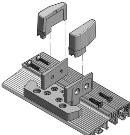
Mittelhalter (MH...) aus Kunststoff inkl. Falzdichtung und Schwelldichtung
